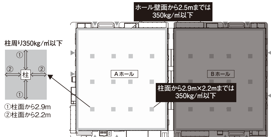
図6. 床耐荷重350kg/m 2 の範囲
